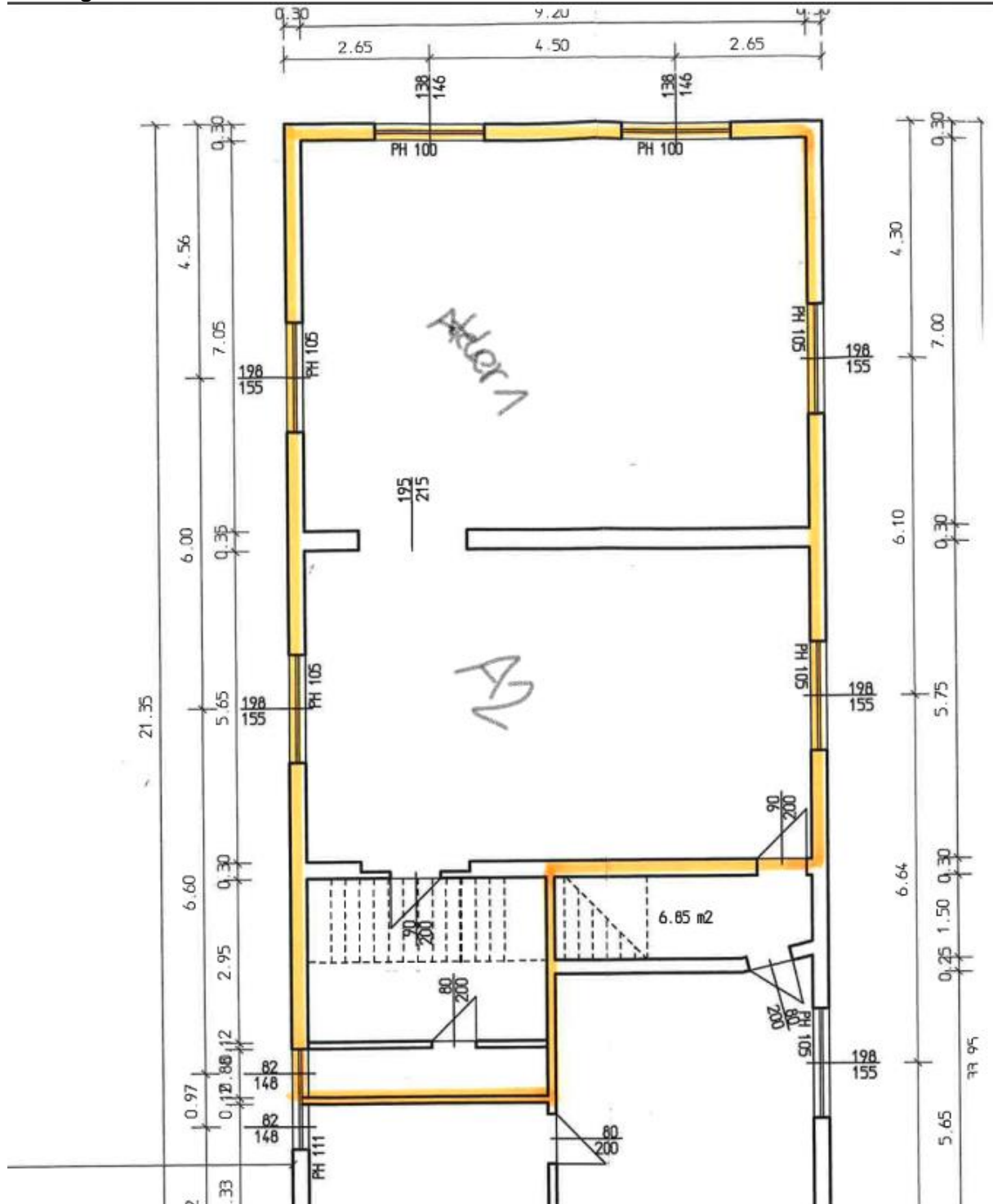
Grundriss Atelier 1
